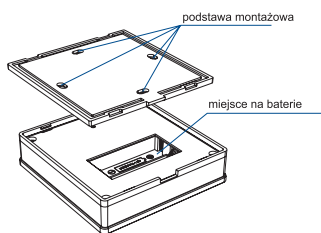
Schemat instalacji w puszcze:
