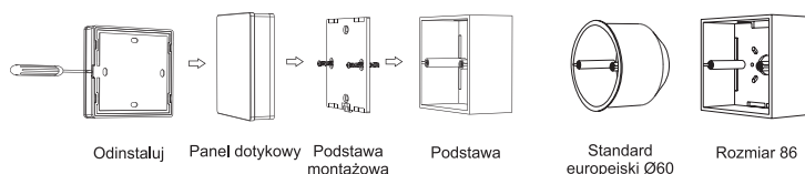
Schemat instalacji w puszcze:
