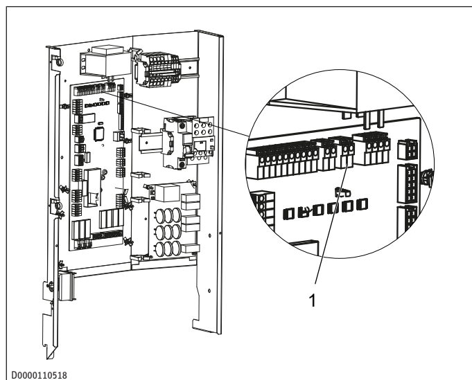
1 T33: Przyłącze czujnika temperatury zewnętrznej
