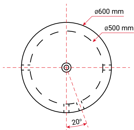
Rzut z przodu
