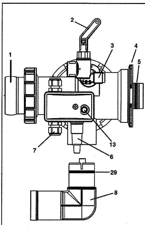
Bild 2: Grundeinheit Draufsicht
