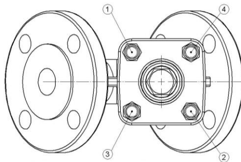
Kolejność dokręcania nakrętek łączących pokrywę z korpusem.
