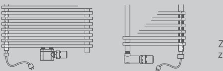
Zestaw VHX-DUO (prosty) z grzałką standard
