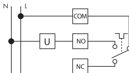
Schemat połączeń / wyprowadzeń
