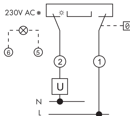
Schemat połączeń / wyprowadzeń
