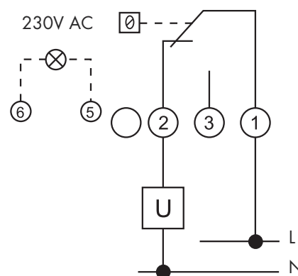
Schemat połączeń / wyprowadzeń
