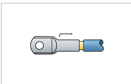
1.1 - Właściwy kierunek i kolejność zaprasowywania końcówek rurowych
