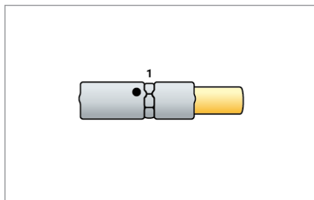
2.2 – Pierwsze zaprasowanie (wewnątrz)
