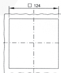
Otwór instalacyjny
