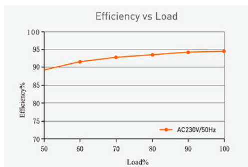
wydajność vs obciążenie / efficiency vs load
