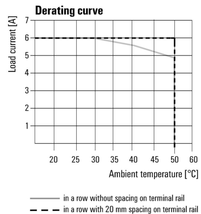
Krzywa obciążalności prądowej
