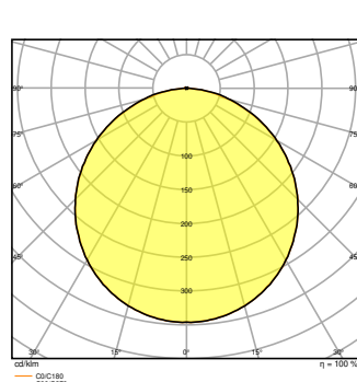
PL CMFT 600 P 33W 865 PS
