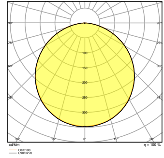
PL CMFT 600 P 30W 865 PS
