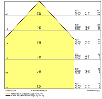
PL CMFT 1200 33W 830 U19 PS EM CONVERSION BOX
