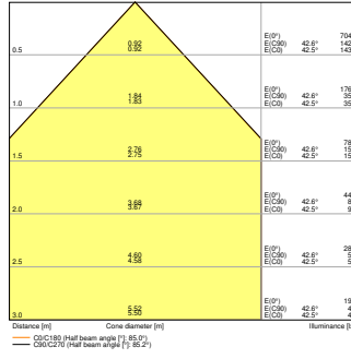
PL CMFT 1200 28W 830 U19 PS
