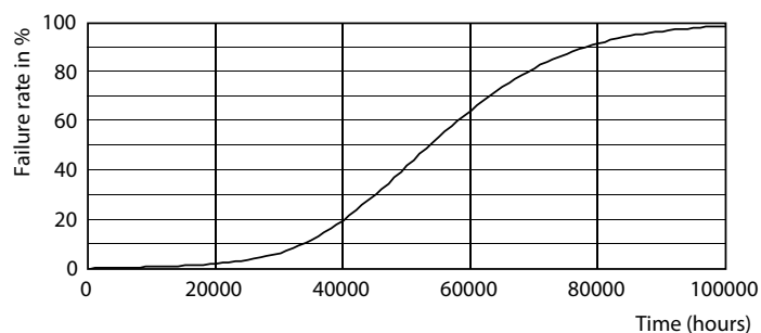
26W G5
